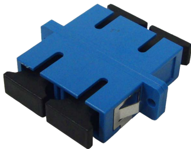
SC Duplex
